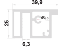
RK-1506 KÜPEŞTE 0,856 kg/m
