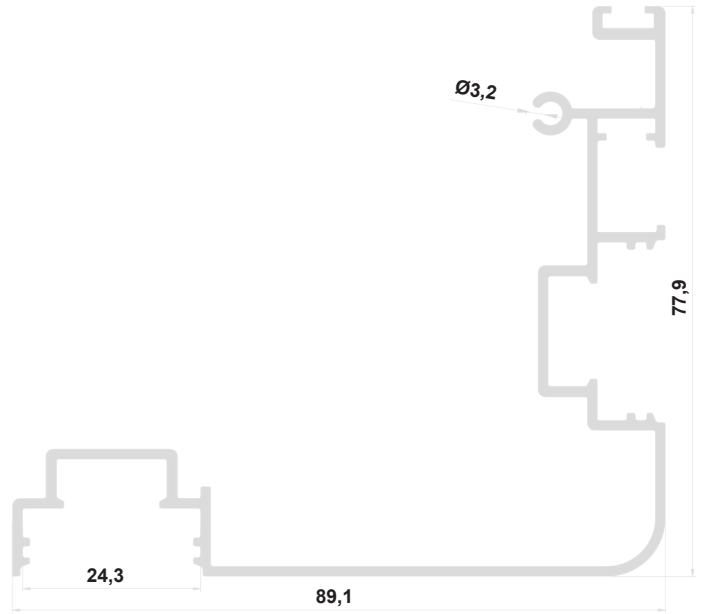
RK-1413 YAN DİKME KAPAK 1,019 kg/m
