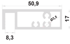
RK-1505 SABİT BAZA 0,851 kg/m
