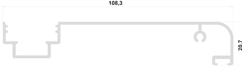
RK-1412 YAN DİKME DIŞ KAPAK 0,69 kg/m
