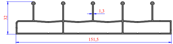
TRS - 3588 1,510 kg/m Yeni Sürme 5'li Alt Ray
