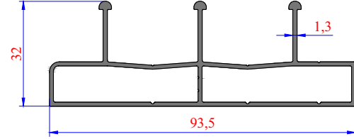
TRS - 3738 0,942 kg/m 3'li Alt Ray
