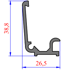
TRS - 3683 0,449 kg/m Sürme Kilit 2
