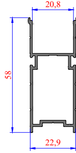
TRS - 3772 0,548 kg/m Isı Camlı Sürme Çekme Kol
