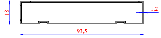
TRS - 3739 0,723 kg/m 3'li Sürme Kutu
