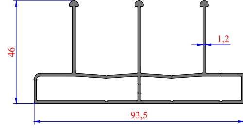
TRS - 3737 1,066 kg/m 3'li Üst Ray
