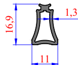
TRS - 3810 0,164 kg/m Sürme Çekme Kulp
