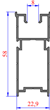
TRS - 3773 0,620 kg/m 8mm Sürme Çekme Kol
