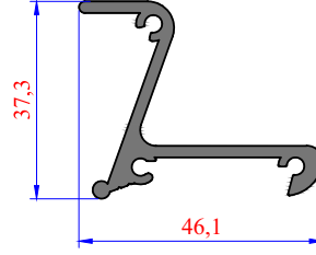
TRS - 3682 0,698 kg/m Sürme Kilit 1
