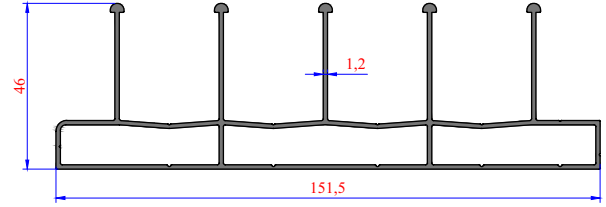
TRS - 3587 1,716 kg/m Yeni Sürme 5'li Üst Ray
