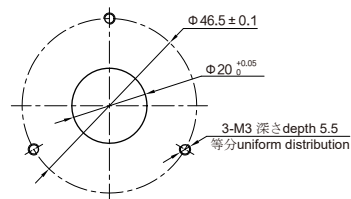
オプション サーボマウント用取付ツメ Options : servo mount fixing nail
