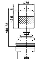
Z軸に1つの押しボタンスイッチ付 Z axis with 1 push button switch
