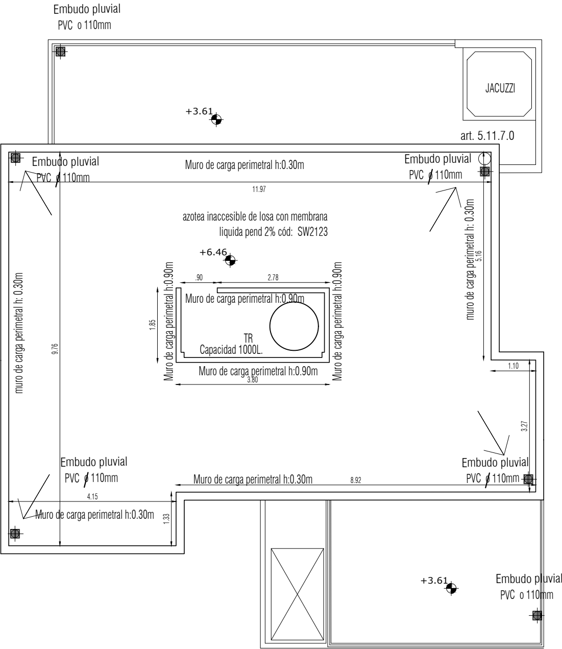
PLANTA TECHOS - ESC.1:50
