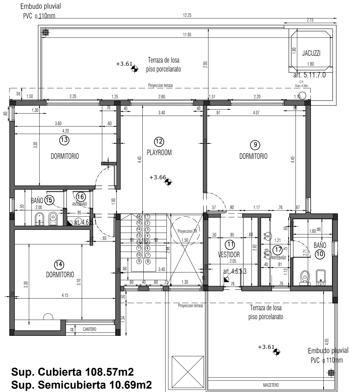
PLANTA ALTA ESC 1:50
