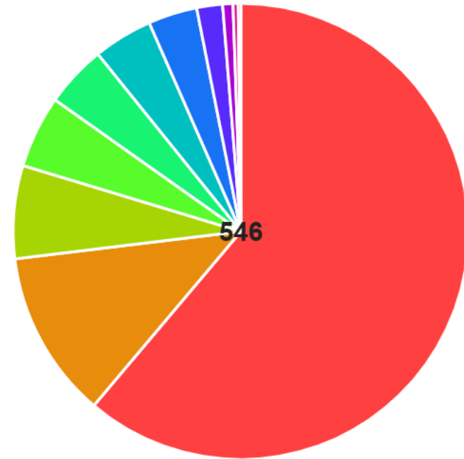
Disposition Codes
