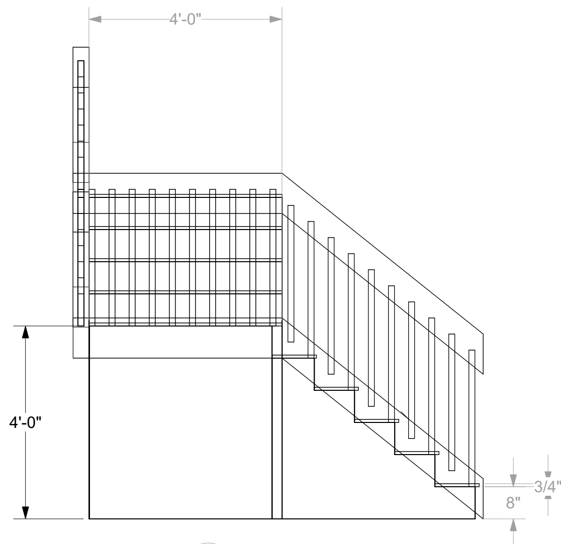
3 Left Side Scale: 1/2" = 1'-0"
