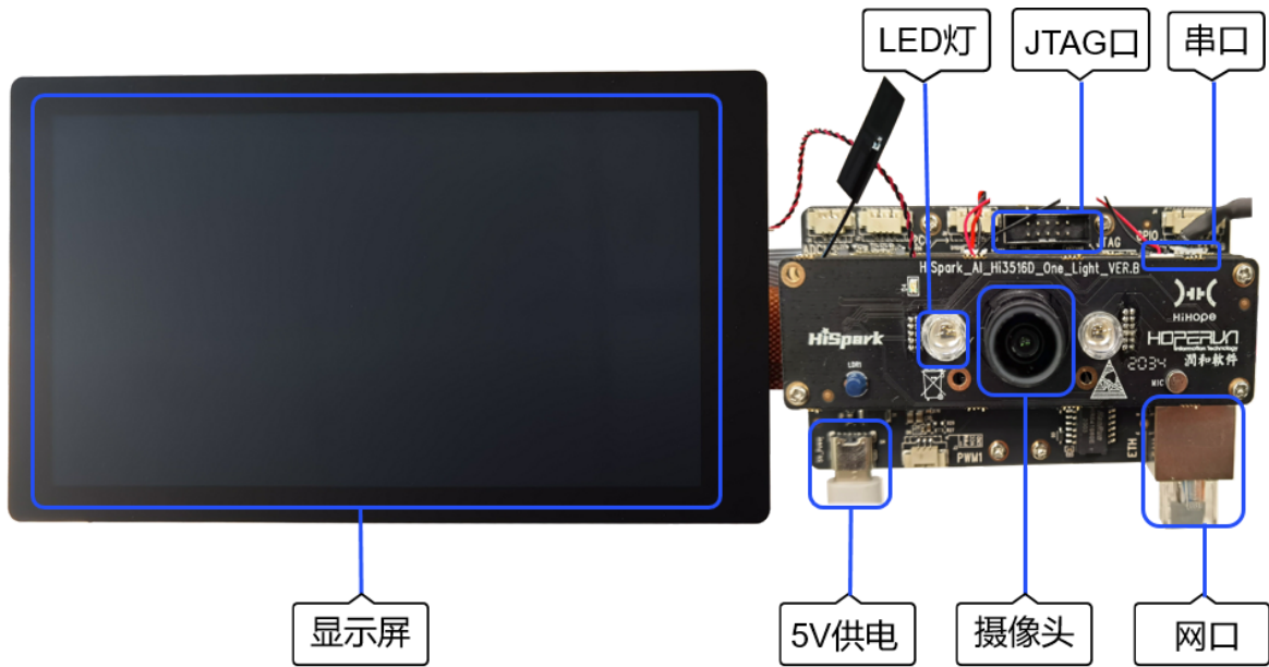
图 1 Hi3516单板正面外观图
