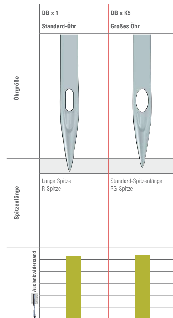
Gegenüberstellung der Nadelsysteme DB x 1 und DB x K5
