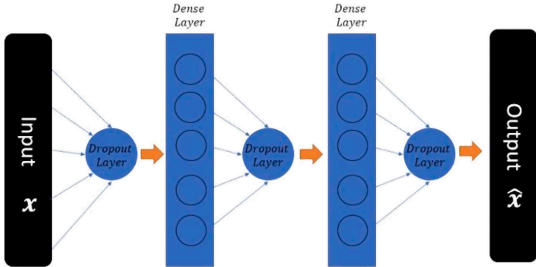
Fig. 4. DANN Schematic.
