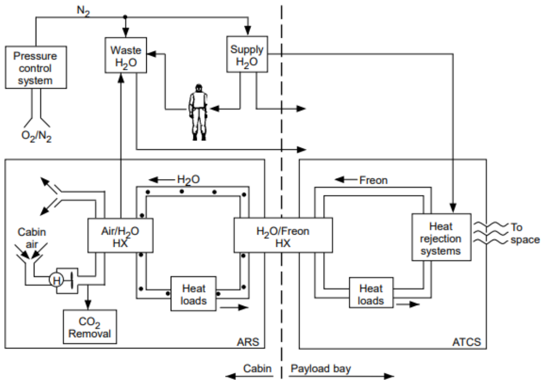
ECLSS OVERVIEW
