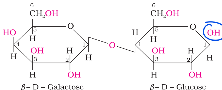
Lactose
