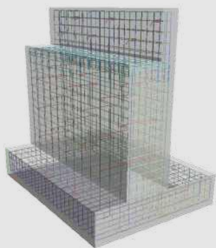
橋台構造
