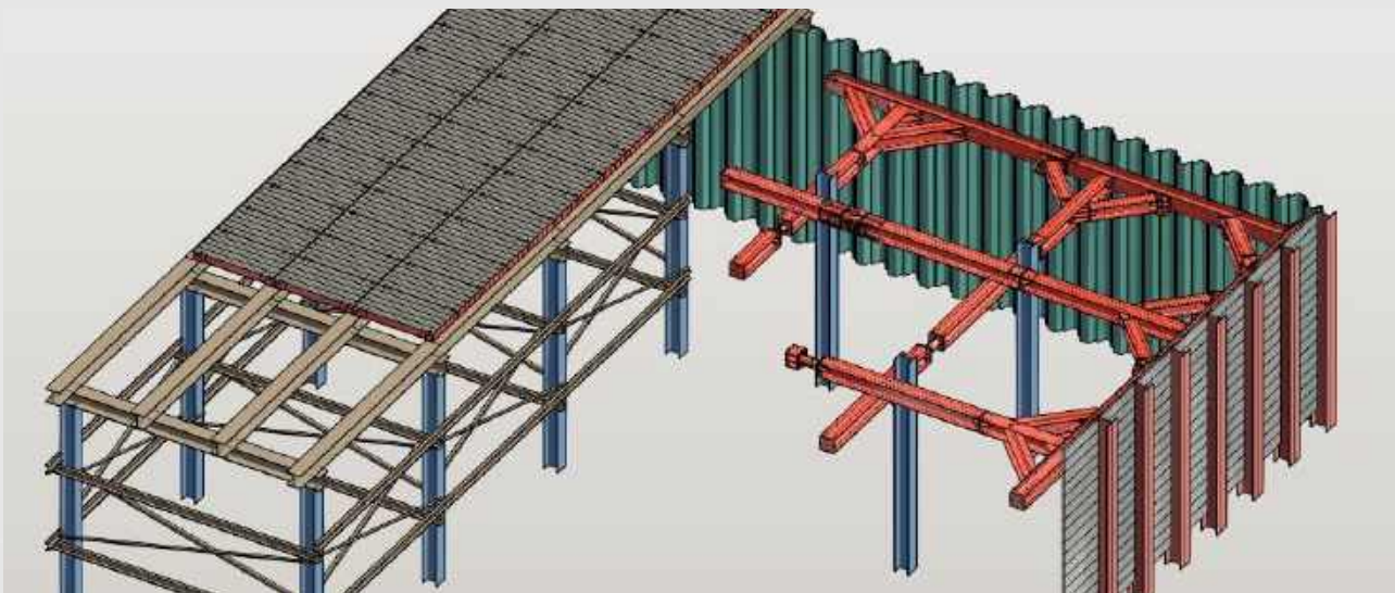
山留工事設計
