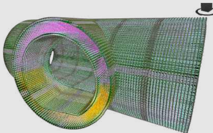
推進工構造
