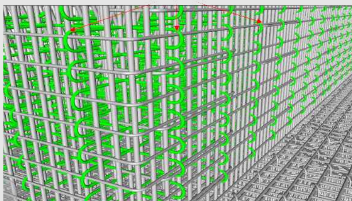
鉄筋干渉チェック
