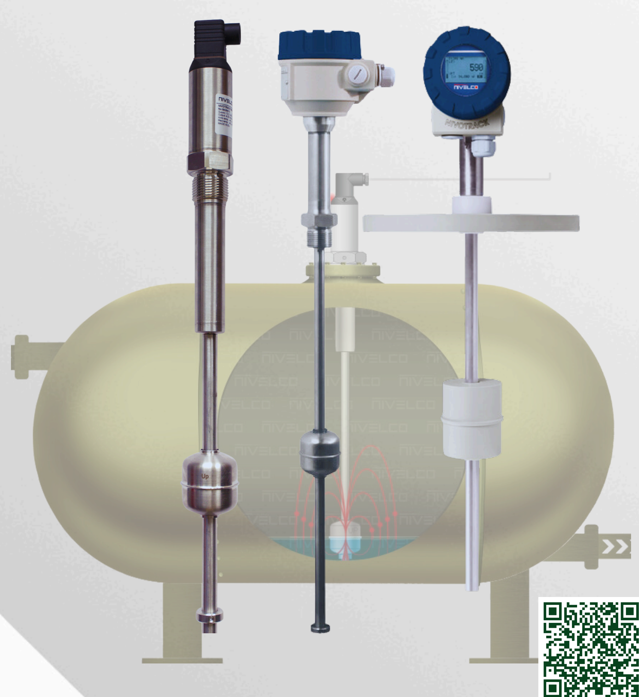
TRANSMISOR DE NIVEL TIPO MAGNETOESTRICTIVO NIVOTRACK
