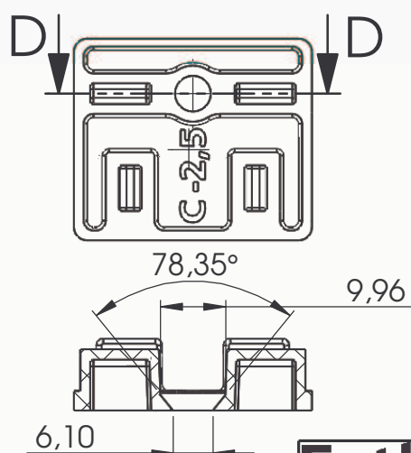
SECTION D-D SCALE 1 : 1
