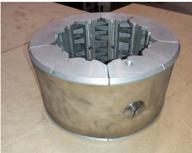
SERVIZIO SOSTITUZIONE FASCE - EXPANDING CHUCK RE-BELTING
