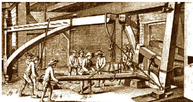
Fabricación de anclas
