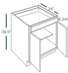
BASE DOUBLE DOOR B24 B30 B36 B27 B33
