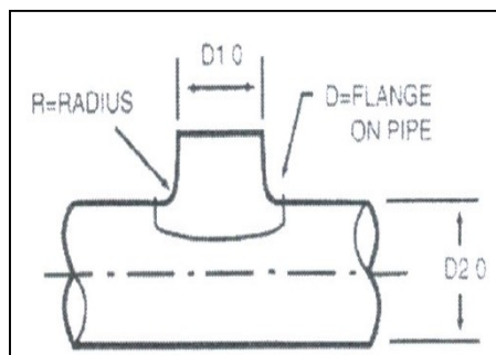
DC - TAP 45° OR 90° TAP
