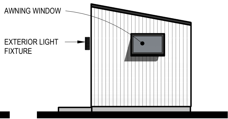
RIGHT ELEVATION
