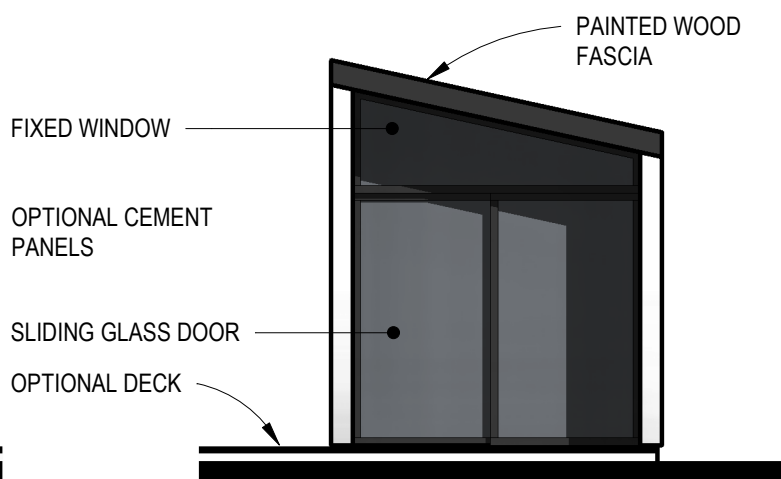
RIGHT ELEVATION
