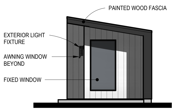
RIGHT ELEVATION
