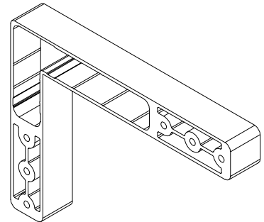
GIUNTO PER MONTANTE CERNIERA HINGE PROFILE JOINT
