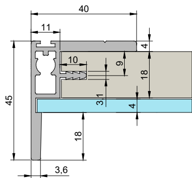
HAND13 - MANIGLIA CON VETRO HANDLE WITH GLASS P10140
