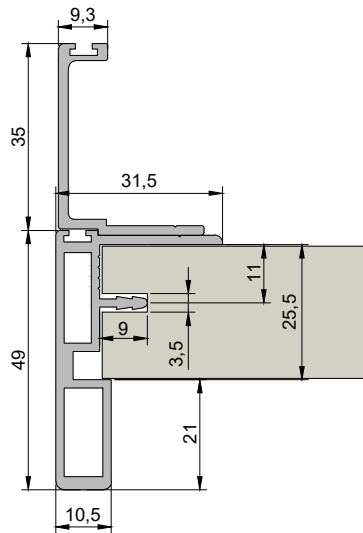
HAND5 - MANIGLIA + PROFILO DI CHIUSURA HANDLE WITH SIDE CLOSING M2024+SC3007
