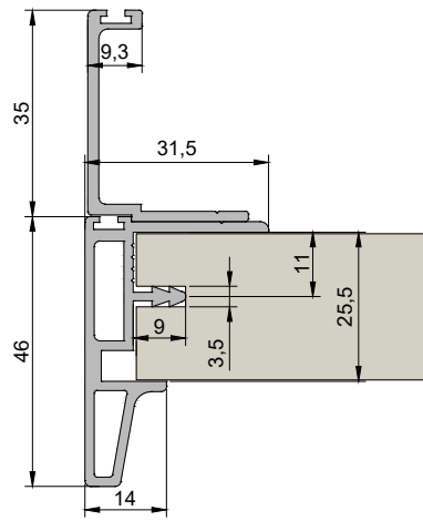
HAND4 - MANIGLIA + PROFILO DI CHIUSURA HANDLE WITH SIDE CLOSING M2022+SC3007
