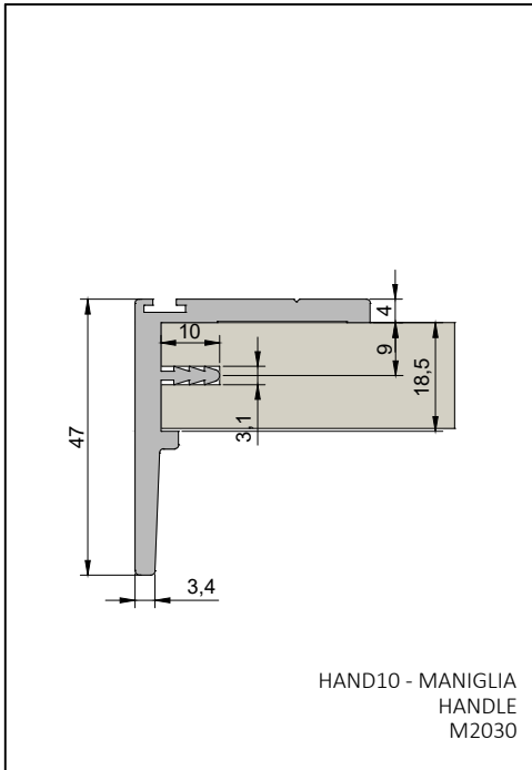
HAND8 - MANIGLIA / CONTROMANIGLIA HANDLE / COUNTER HANDLE M2028
