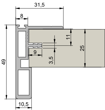
HAND5 - MANIGLIA HANDLE M2024
