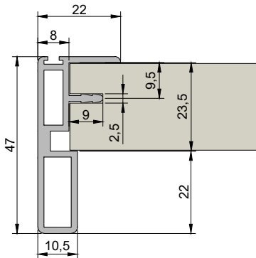
HAND6 - MANIGLIA HANDLE M2026
