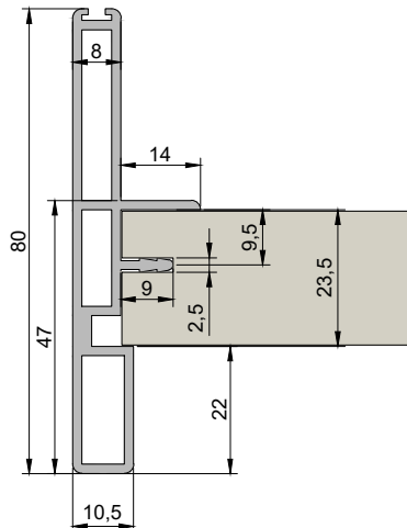
HAND6 - MANIGLIA ALTA HIGH HANDLE M2025
