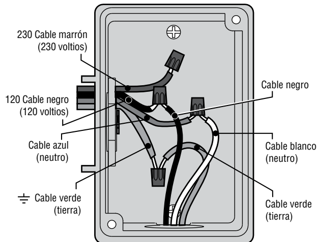
Caja de conexiones sin regleta de terminales (120 voltios)
