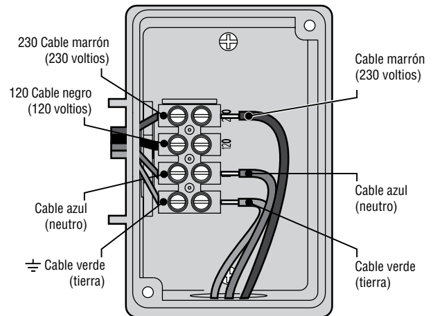
Caja de conexiones con regleta de terminales (230 voltios)
