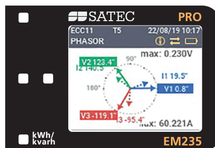
Pantalla Fasorial
