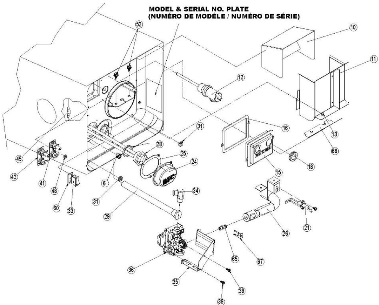
REAR VIEW (VUE DE L'ARRIERE)
