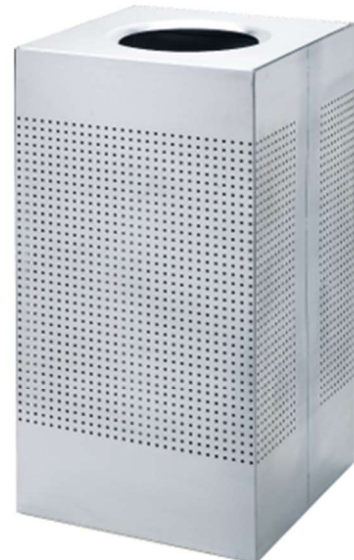
NDA-207 方形冲孔垃圾桶 SIZE:A(L)300×(W)300×(H)680mm SIZE:B(L)400×(W)400×(H)760mm
