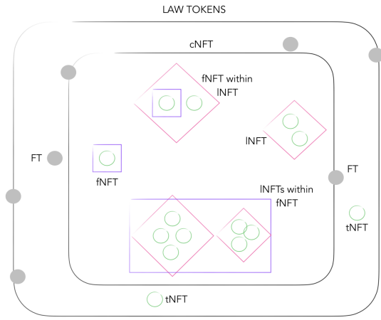
Fig. 3: NFT Wrappers
