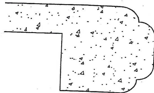
D-310 DOUBLE 1/4" RADIUS B.B.
