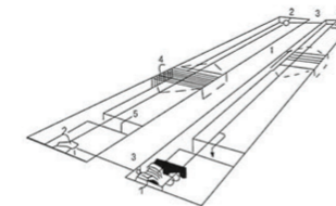
1、主机座 (绞盘) 2、转角轮 3、牵引绳 4、刮粪板 5、横向粪沟
