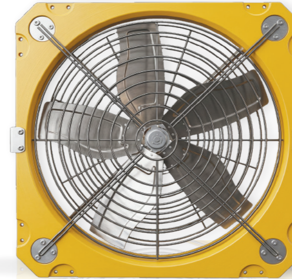
塑料防腐牛舍悬挂式风机
