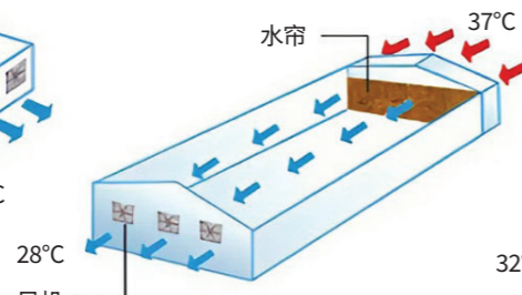
纵向水帘降温系统 Longitudinal cooling pad exhaust fan system
