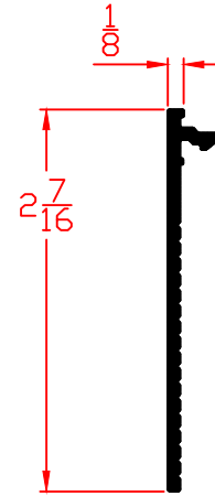
5927 Masonry Flange
