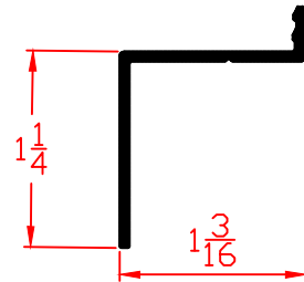
5945 4-9/16" Backset Windbreak
