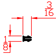
5924 Groove Filler
