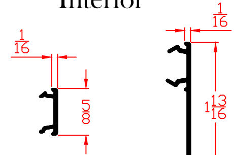
5839 1/2" Groove Filler
