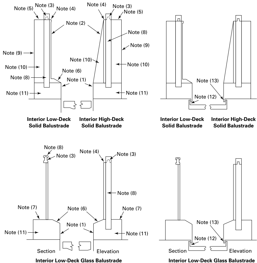
Fig. I-3 Escalator Nomenclature
