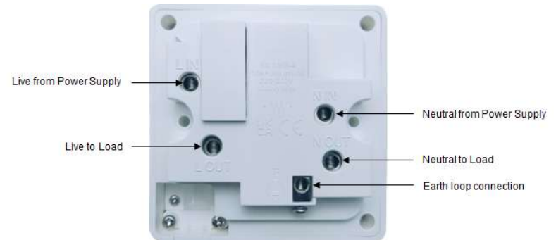
Figuur 1: Bedradingsschema
