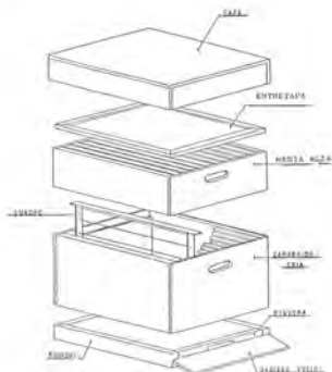
Figura 13.- Despiece de la colmena Dadant.
