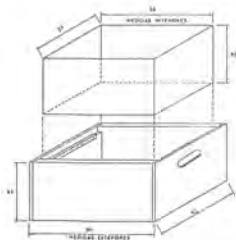
Figura 11.- Dimensiones interiores y exteriores de una colmena Perfección (en cms.)
