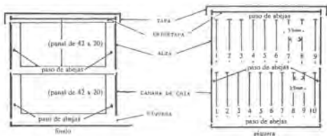
Figura 10.- Sección lateral y frontal de una colmena Perfección.
