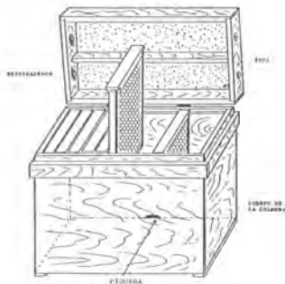
Figura 13.- Colmena Layens.
