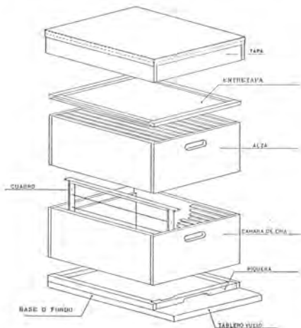
Figura 8.- Despiece de una colmena movlista
