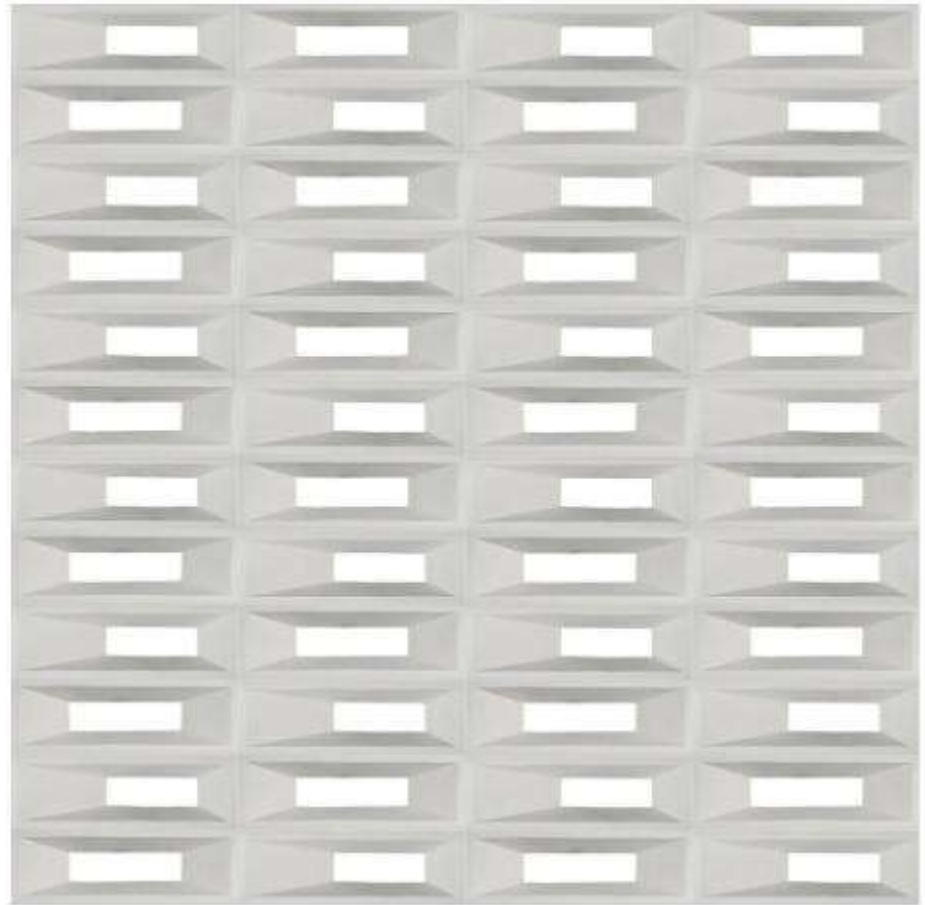
Samahil 60x20x10cm - 14.7kg 8.3pz/m 2
