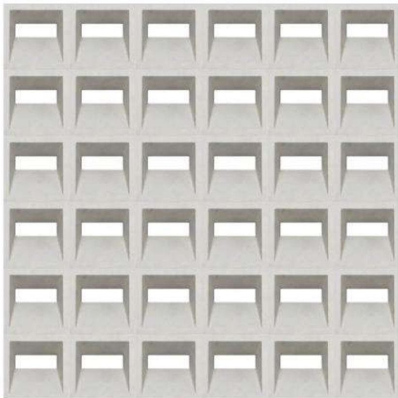
Tekax 20x20x10cm - 4.4kg 25pz/m2
