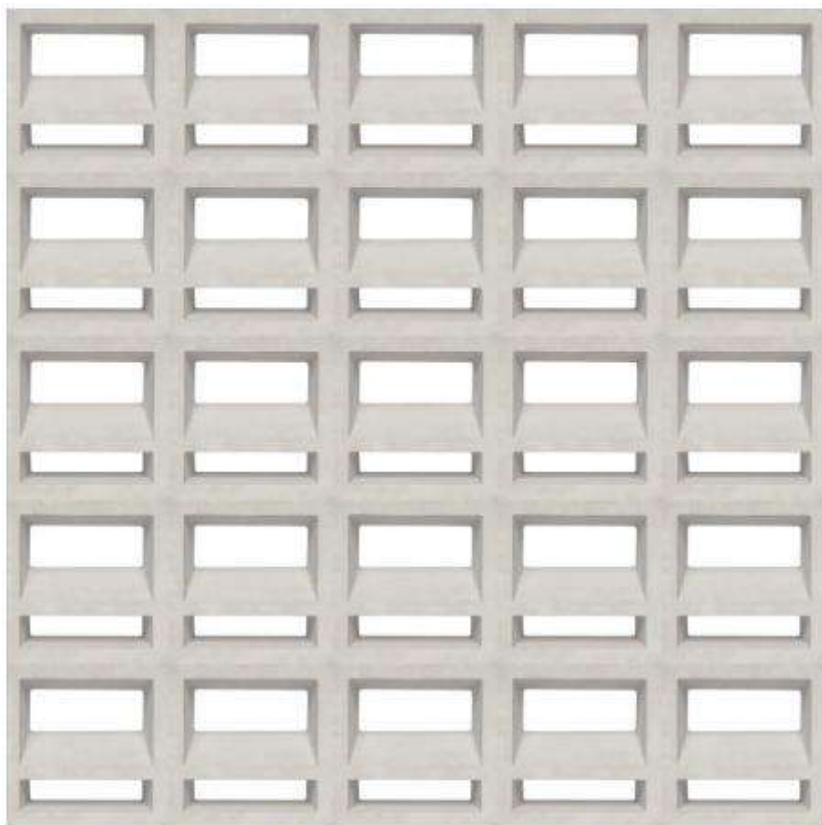
Muna 20x20x10cm - 4.5kg 25pz/m2
