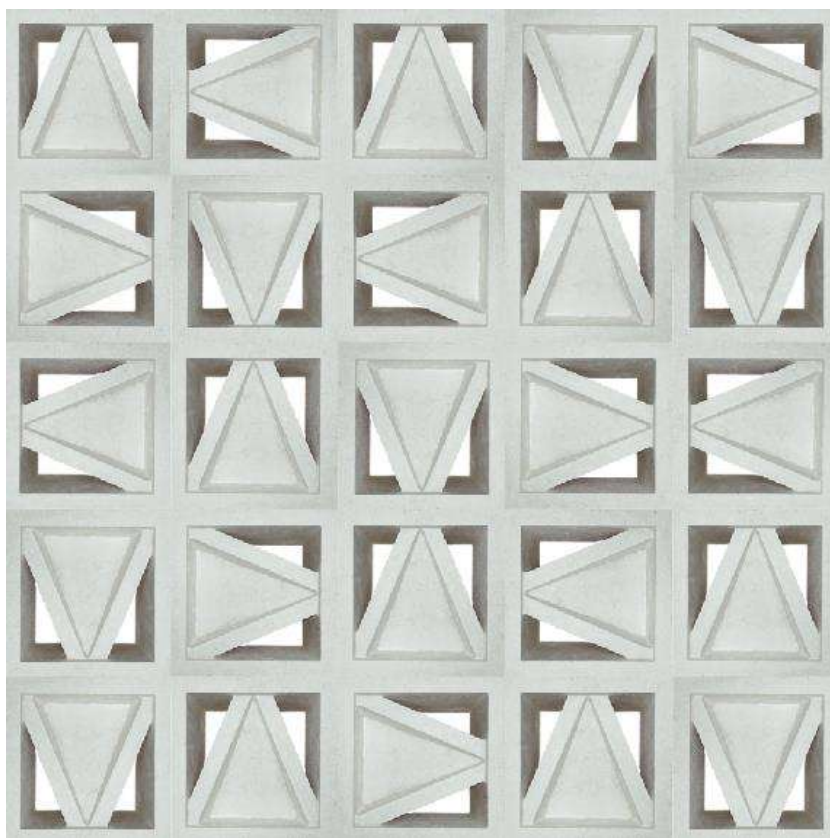
Sacnicté 20x20x10cm - 5.1kg 25pz/m2
