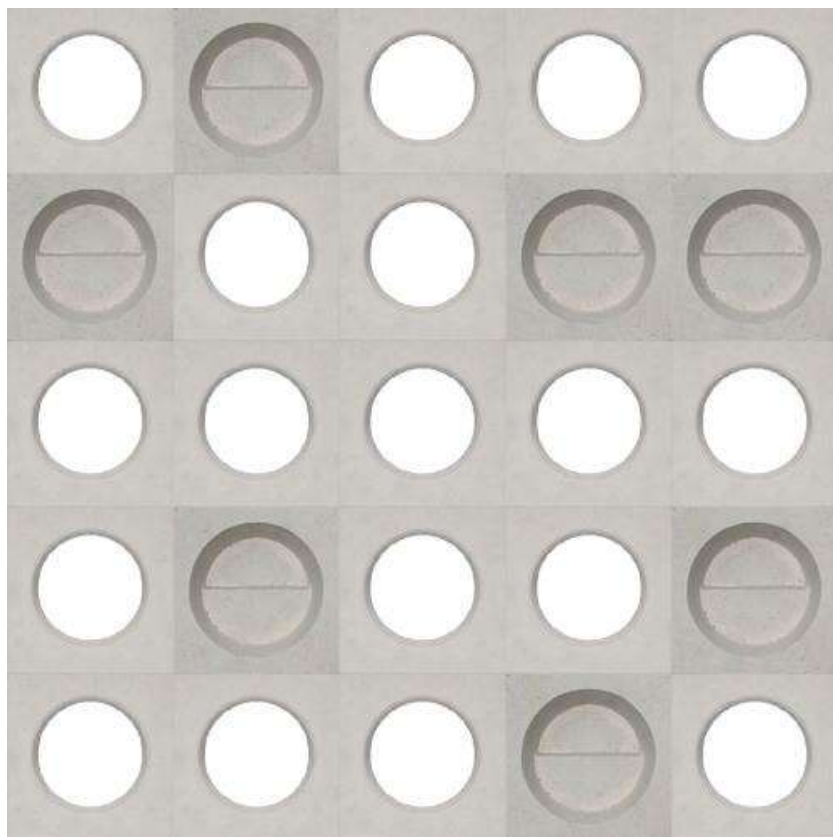
Teka1 20x20x10cm - 5.5kg 25pz/m2
