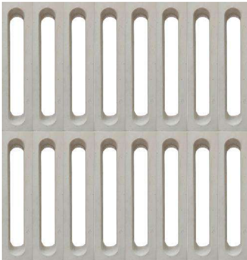
0xkutzcab (doble vista) 40x10x10cm - 3.5kg 25pz/m2
