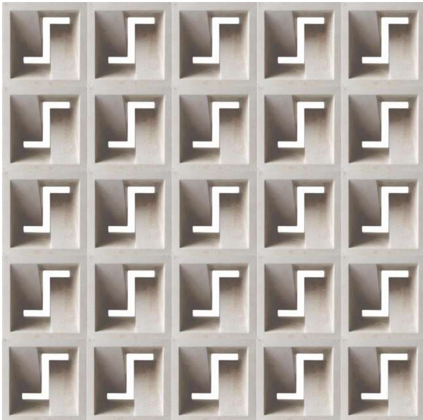
Mayapán 20x20x10cm – 4.6kg 25pz/m 2
