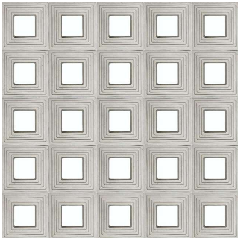
Xcunyá 20x20x10cm - 4.2kg 25pz/m2
