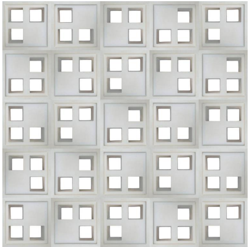
Ekmu1 20x20x10cm - 2.8kg 25pz/m2
