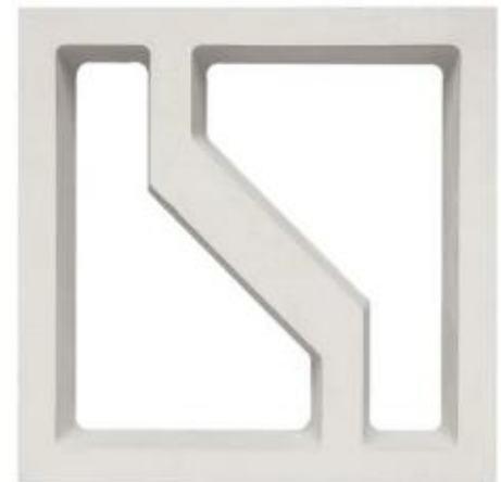
Calotmul 30x30x7cm - 5.3kg 11.1pz/m2
