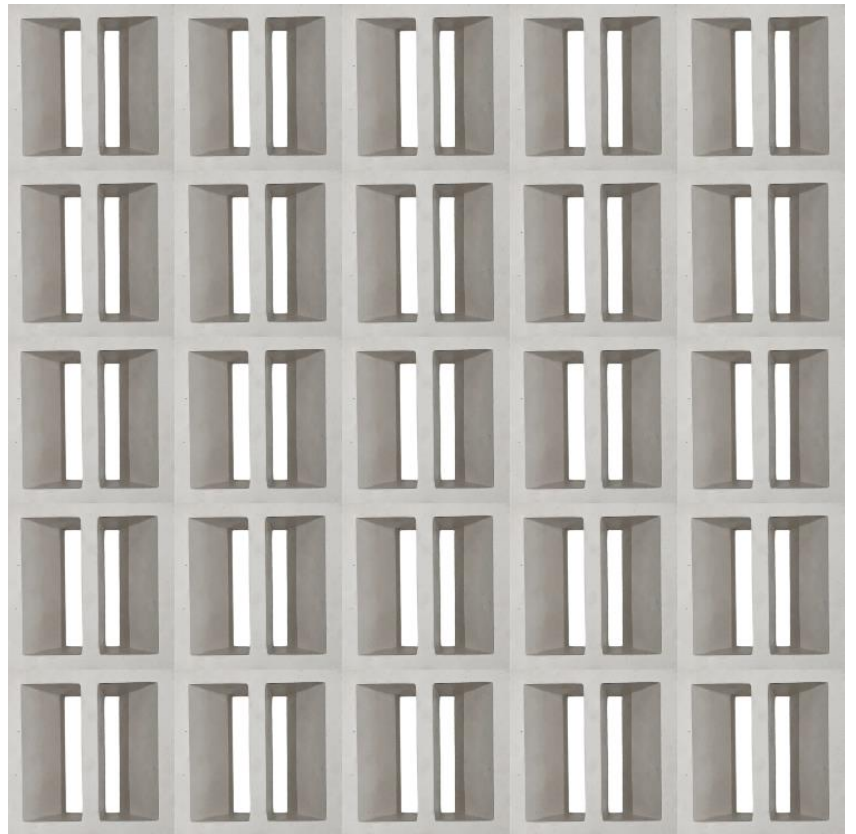
Tixpéhua1 20x20x10cm - 4.2kg 25pz/m2
