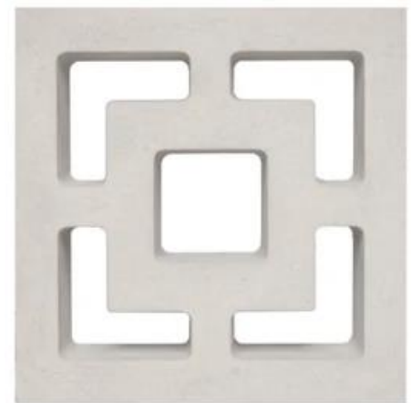
Temozón 30x30x7cm - 7.6kg 11.1pz/m2
