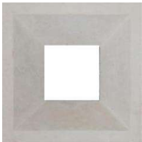
Oncán (doble vista) 20x20x10cm – 4.1kg 25pz/m 2
