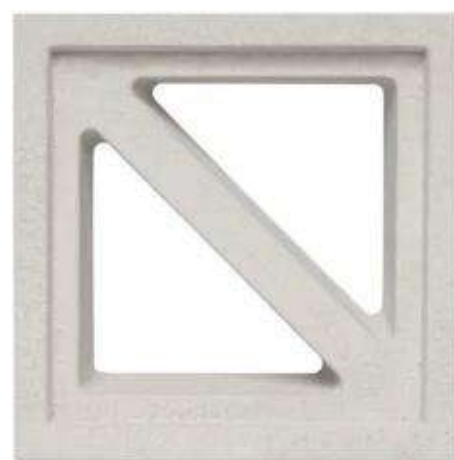
Tekit 20x20x6cm - 2.5kg 25pz/m2
