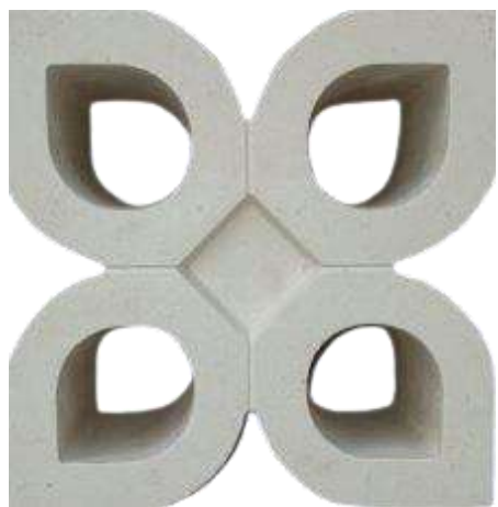
Tunkás 20x20x10cm – 4.7kg 25pz/m 2
