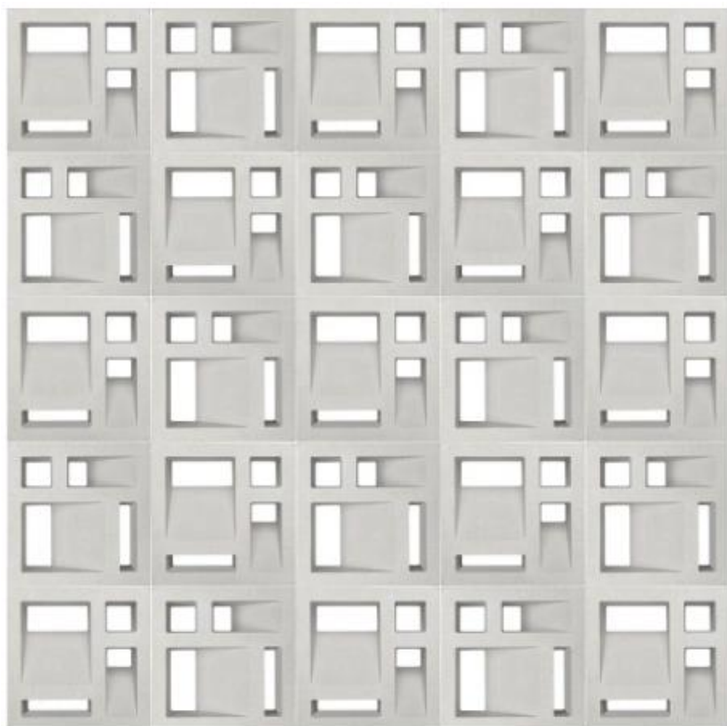
Kinchil 20x20x10cm - 4.6kg
