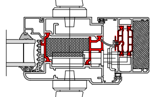
➤ 58BD HI LOCK JAMB
