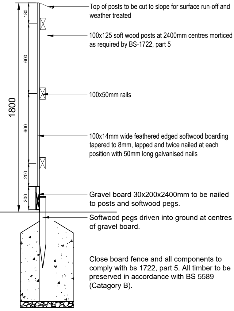
Section A-A
