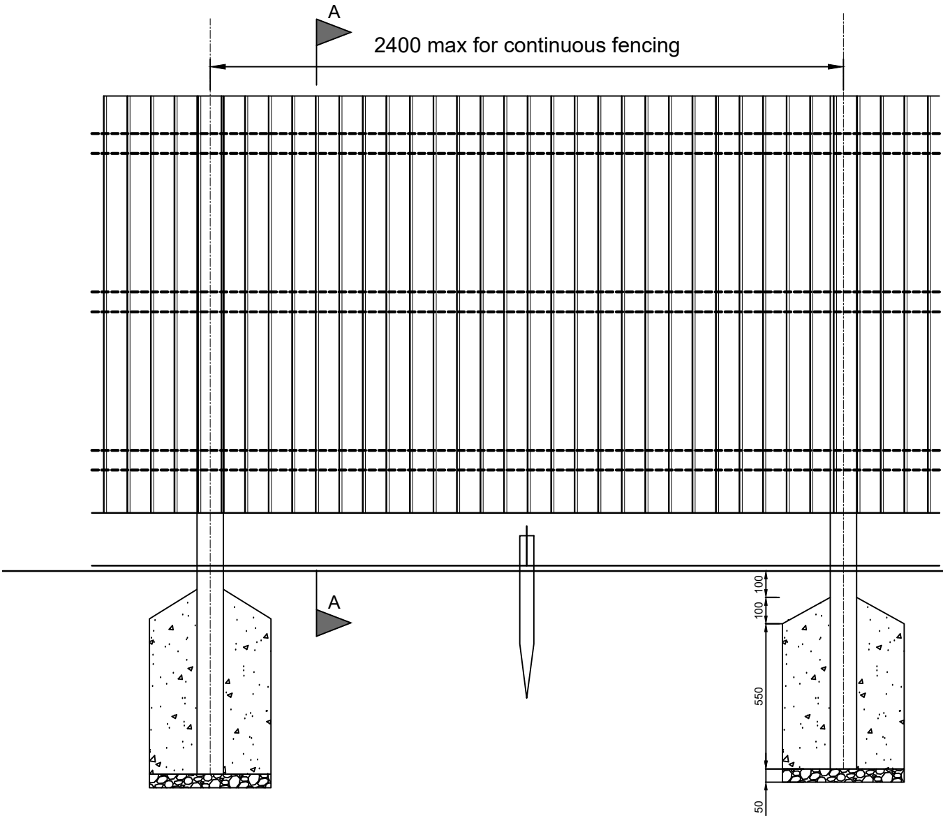
Elevation
