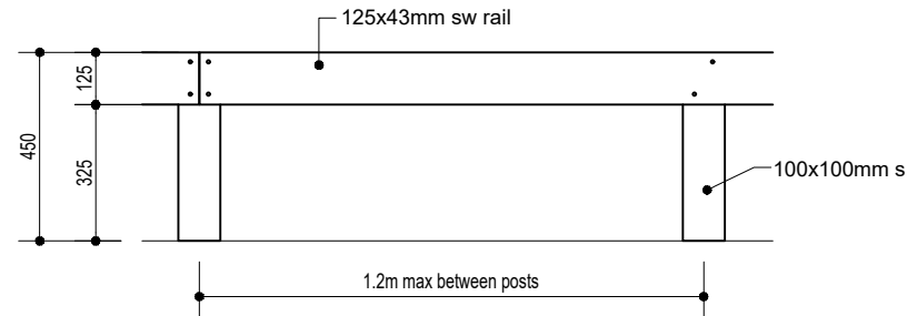
ELEVATION
