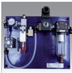
NB1/NB2 Nebulizzatore per la lubrificazione lama ad uno e due ugelli. Sprayer for blade lubrication one/two nozzle. Micro pulvérisation pour la lubrification du ruban à un/deux buses.
