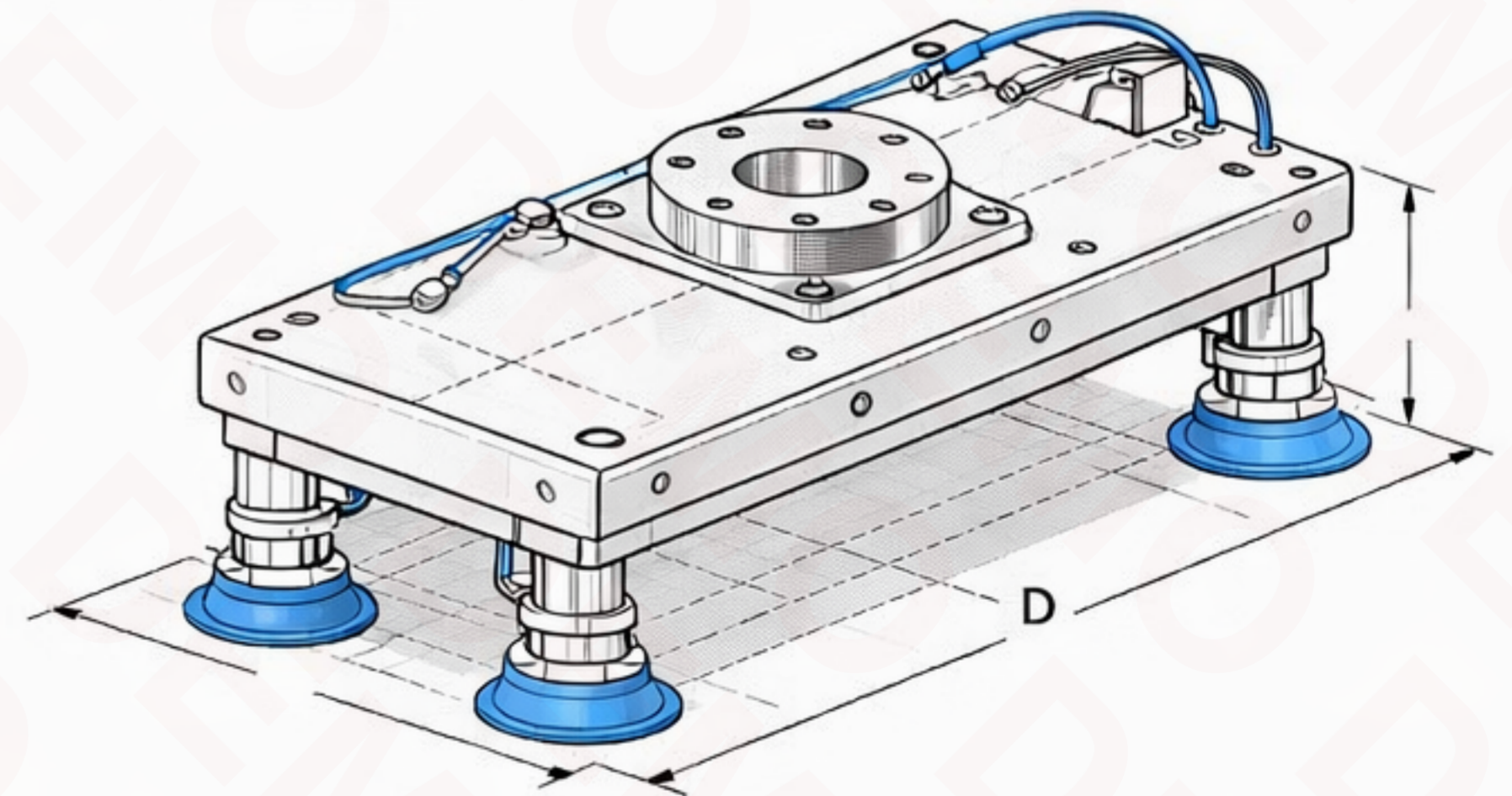
VISTA ISOMÉTRICA
