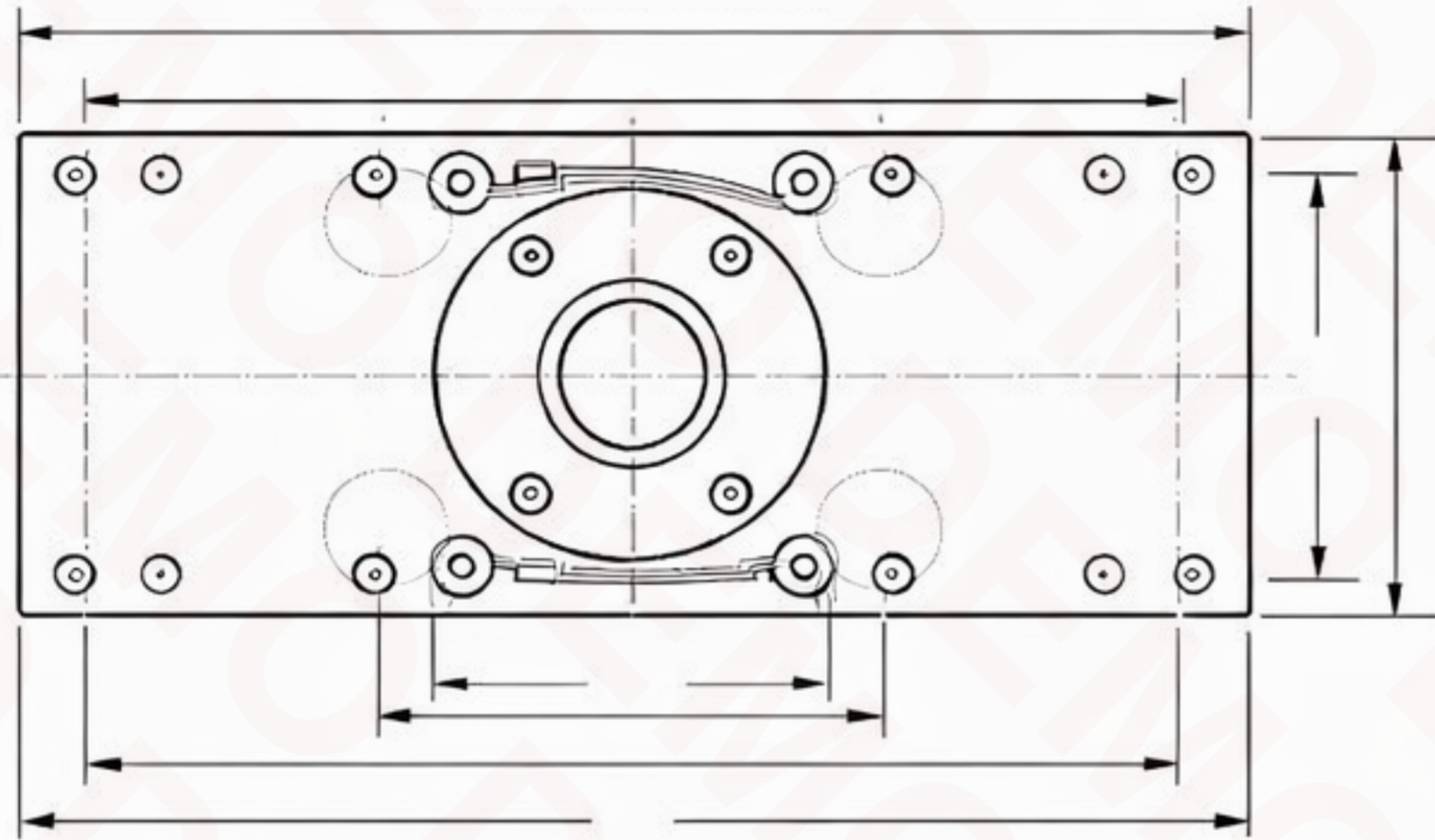
VISTA SUPERIOR
