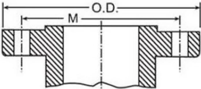
Flange
