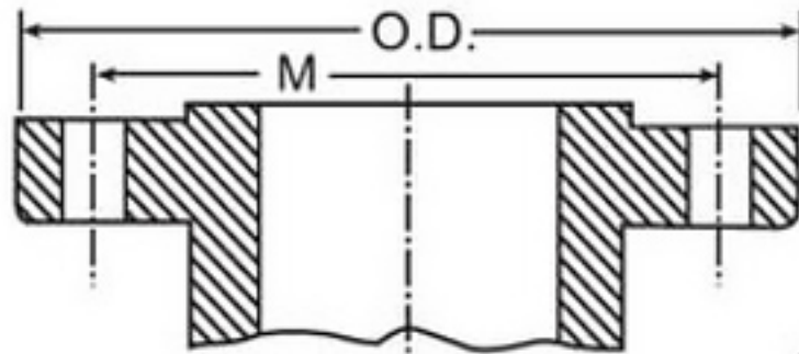
Flange
