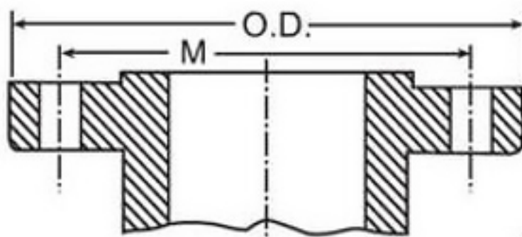
Flange
