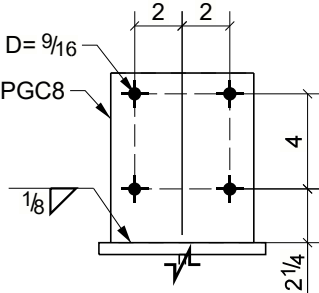
C - C
