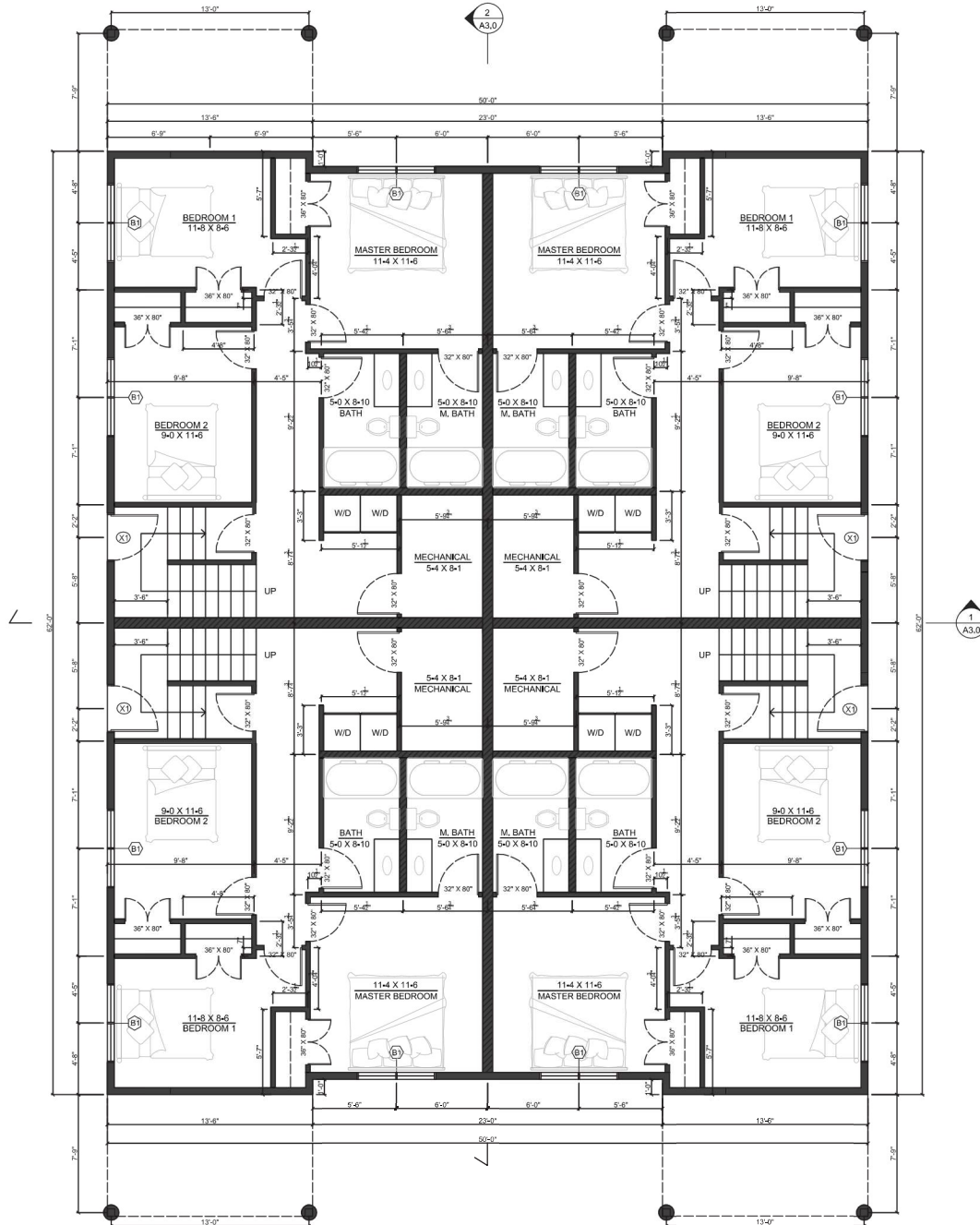
1 A1.2 BASEMENT PLAN SCALE: 1/8" = 1'-0"
